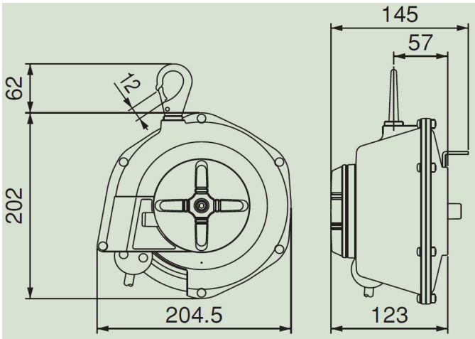
寸法図(外形)
