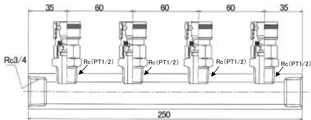
正面図
