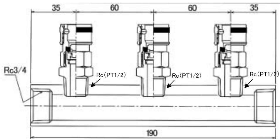
正面図
