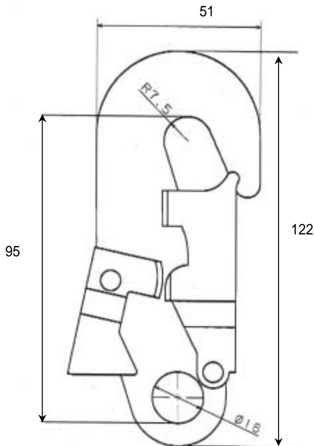
フック寸法図
