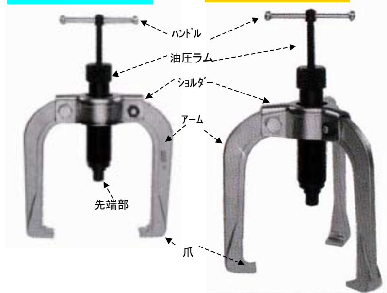
2本爪プーラーセット状態
