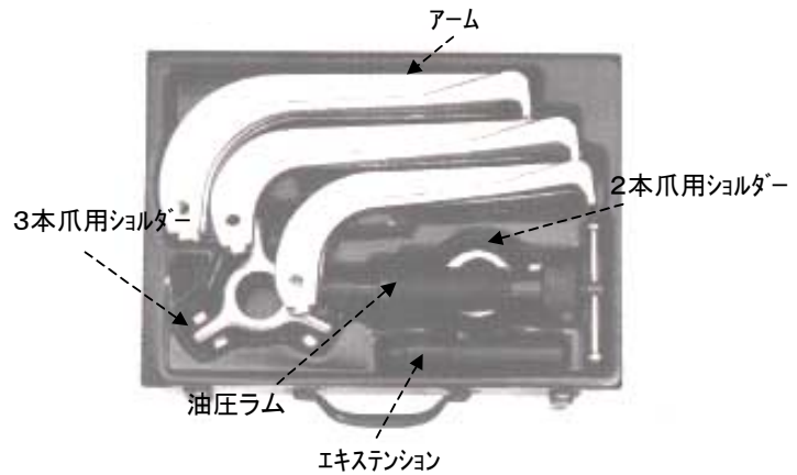
2本爪プーラーセット状態
