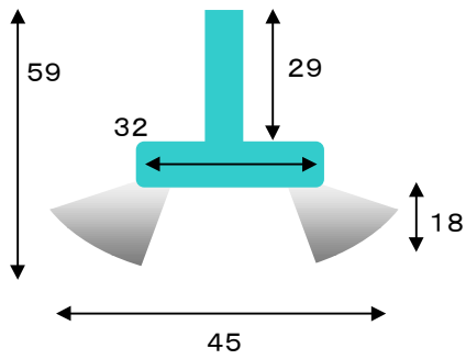
EA819BU-45(断面)
