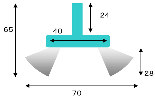
EA819BU-70(断面)
