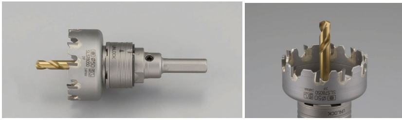
超硬付ホールソーセット(刃+ストレート10mmシャンク+センタードリル)
