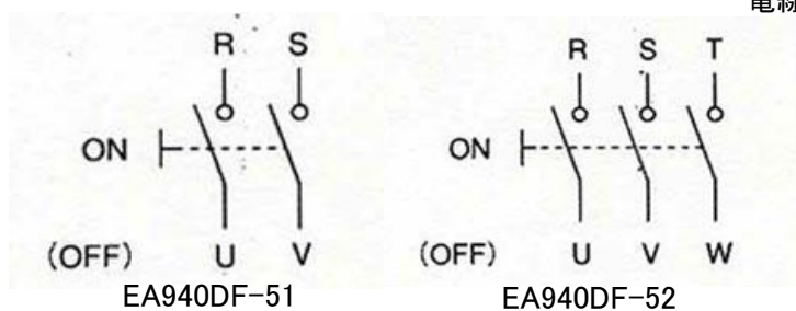
(接点構成表)
