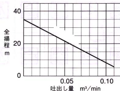
■性能曲線
