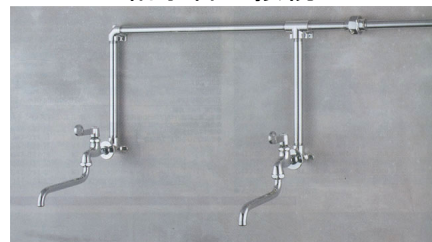
給水管の接続
