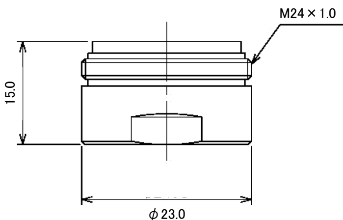
本体サイズ
