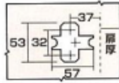
【座金取付け位置】
