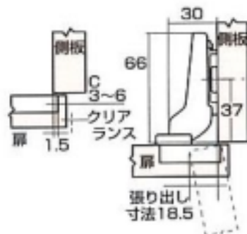
【座金取付け位置】
