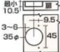
【カップ取付け位置】
