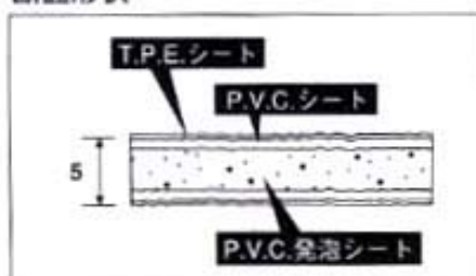
断面形状
