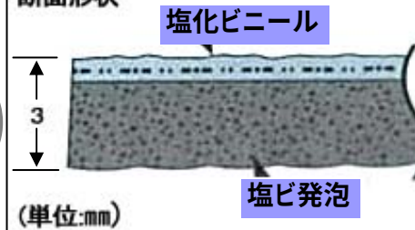
断面形状
