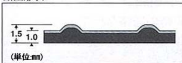
断面形状
