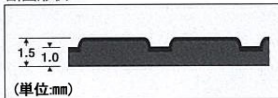
断面形状
