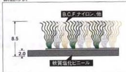
断面形状
