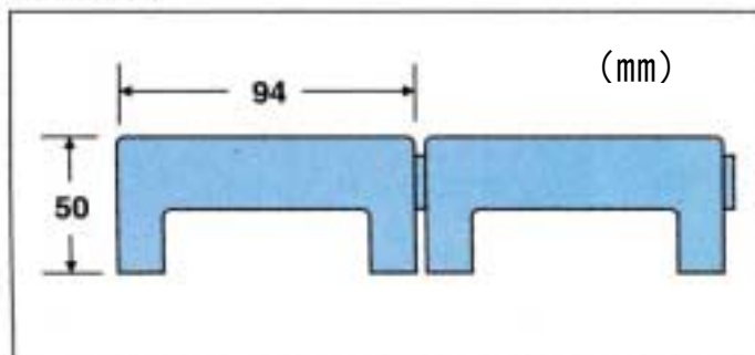
側面形状
