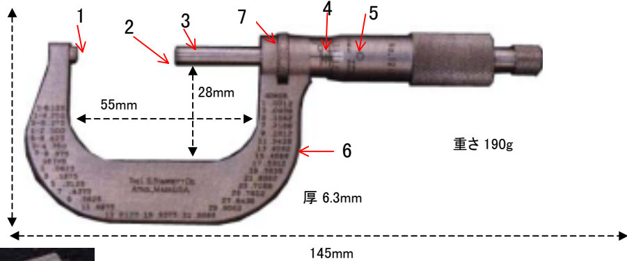
アタッチメント装着状態 (25—50mm間を計測します。)
