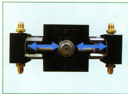
ハイスピード&ハイパワー回収を実現する ツインシリンダー式オイルレスコンプレッサ
