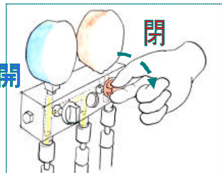
③ 冷媒充填
