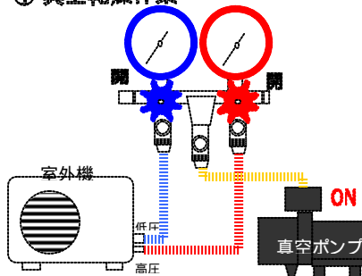
① 真空乾燥作業
