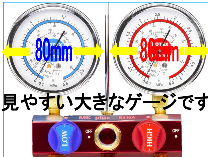
② エアコンの運転圧力計測
