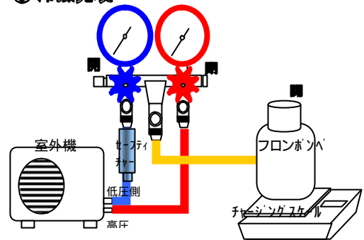
③ 冷媒充填
