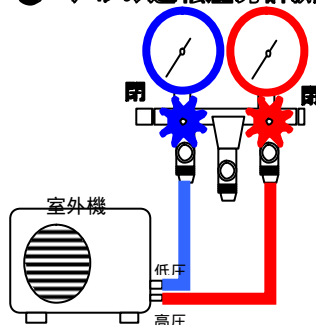
② エアコンの運転圧力計測
