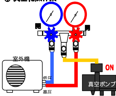
① 真空乾燥作業
