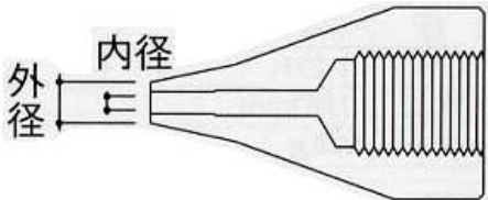
標準ノズル: 内径: φ1.0、外径: φ2.0
