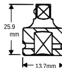
1/4" × 3/8" アダプタ
