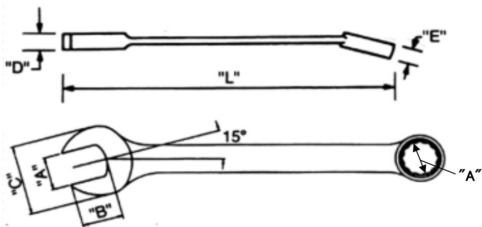
セット構成品寸法
