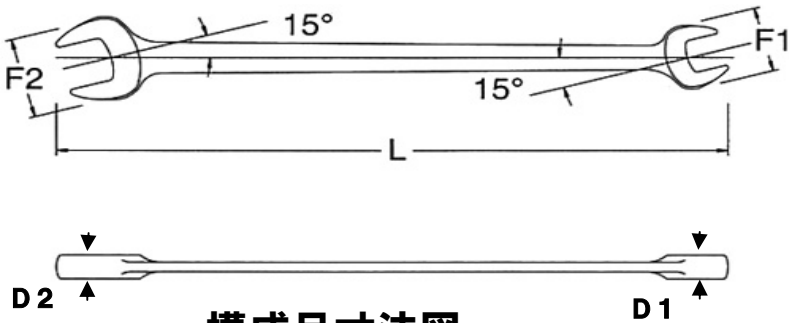
構成品寸法図
