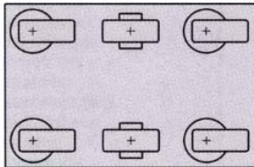
○ スイベルキャスター×4 固定キャスター×2 経済的とはいえないが重量物及び長距離に。プレーン保持
